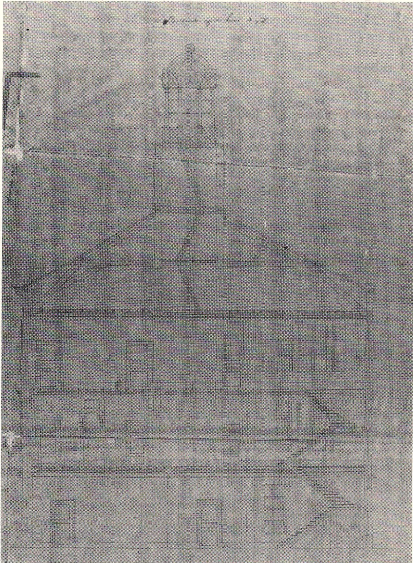
Illustratie 5: Deze doorsnede van Roelandts ontwerp (1828) laat zien hoe de trap-partij als blikvanger fungeert op elke verdieping en tegelijk het bindend element vormt in zijn stadhuisontwerp (GENT, UNIVERSITEITSBIBLIOTHEEK).
